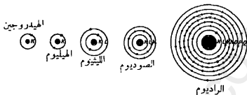
الشكل ٢ - تكوين الذرات الألكتروني
