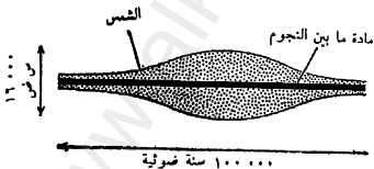
الشكل ٨ - المجرة
