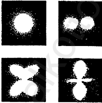
شكل ٣ . - الذرة حسب الميكانيكا التوجيهية
