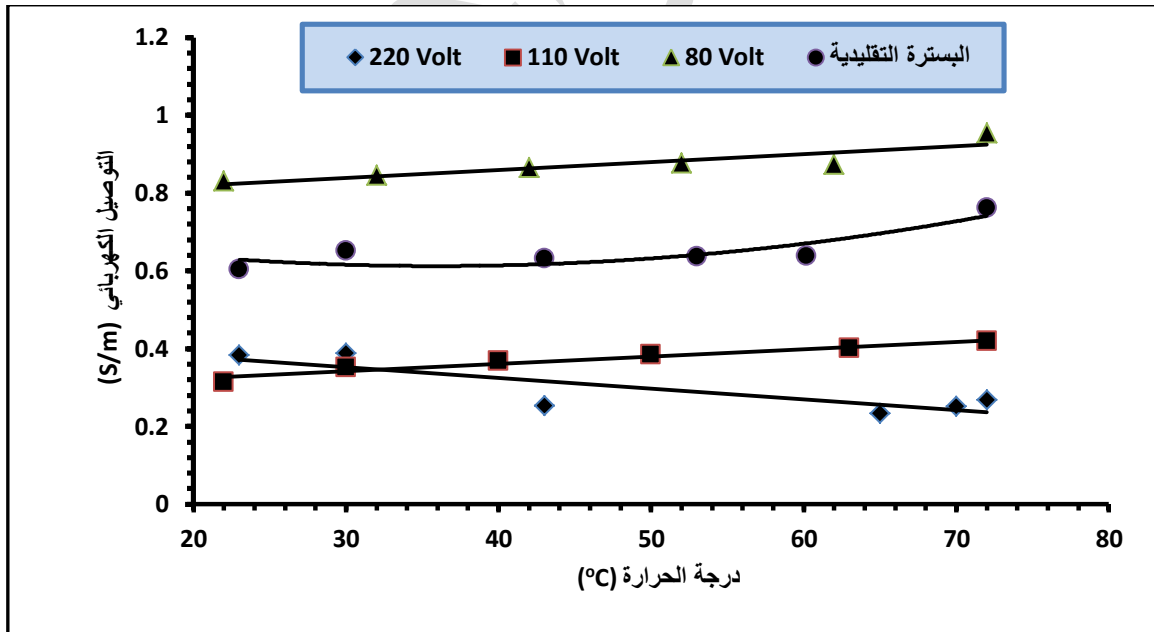
شكل (3) : العلاقة بين التوصيل الكهربائي ودرجة الحرارة لفرق الجهد 220 V ، 110 ، 80 ، والبسترة التقليدية السريعة
