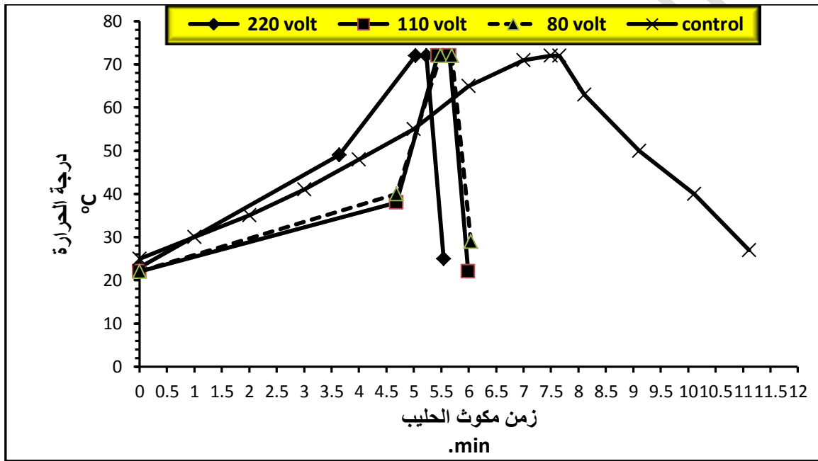
شكل (7) : العلاقة بين درجة الحرارة وزمن مكوث الحليب في جهاز التسخين الاومي لفروق الجهد 220 V ، 110 ، 80 والبسترة التقليدية السريعة
