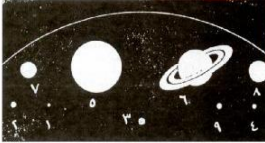
• النسبة بين أحجام الكواكب والشمس
