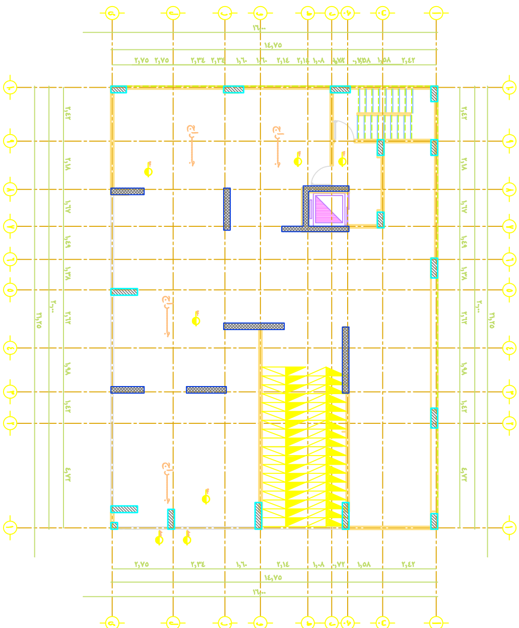
مسقط افقى للبردروم
