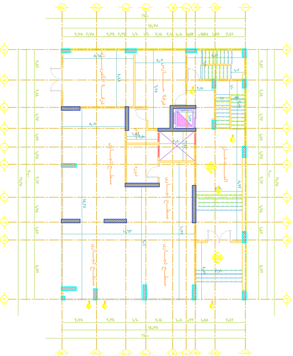
مسح قضا افقى للدور الارضى
