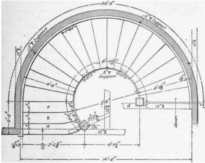
السلالم الهندسية ذات البئر المفتوح .
