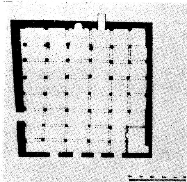
شكل 27 - مخطط جامع قسطنطينية.
