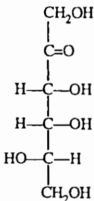
L—Tagatose
