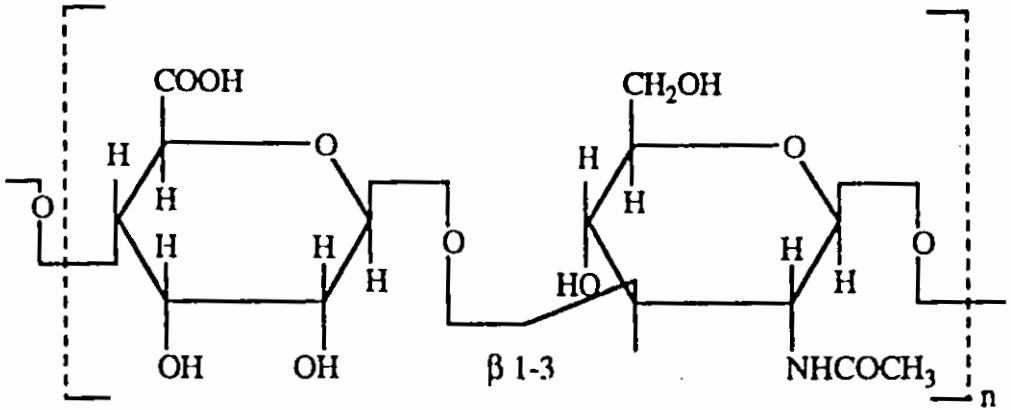
الوحدة البنائية لحامض الهيايورك
