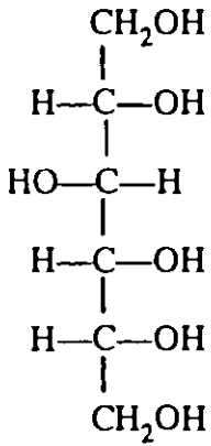
D—Sorbitol
