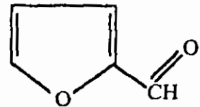
الفورفورال
