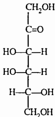
D—Tagatose
