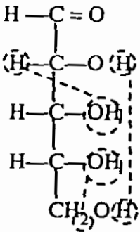
سكر خماسي Pentose
