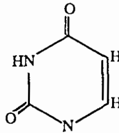
اليوراسيل Uracil 2,4 داي أكسي بيريميدين 2,4 Dioxy rimidne Pyrimidine
