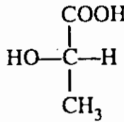
L-Lactic
