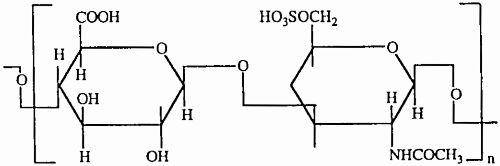
الوحدة البنائية للـ Chondroitin sulfate
