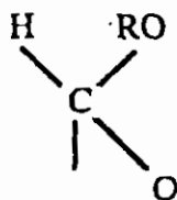
\alpha -O-glycoside ألفا-O- كلايكوسايد
