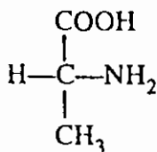
D-Alanine (D) الالين
