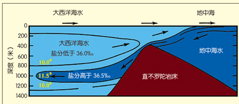
图13：地中海的海水，从直布罗陀海底山脊的上方进入大西洋后仍能保持其本身温暖、含盐及低密度的特质，是因为这条界限将它们隔开。温度以摄氏表示（ ^{\circ} ）。（ Marine Geology [海洋地质学]，作者昆宁 (Kuenen)，第 43 页，稍有修改。）
