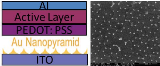
شكل رقم (٧-٥) الشكل الهرمي لجسيمات الذهب التي استخدمت، لدراسة تأثيرها البلازموني في كفاءة الخلية الكهروضوئية العضوية (٩٤).
