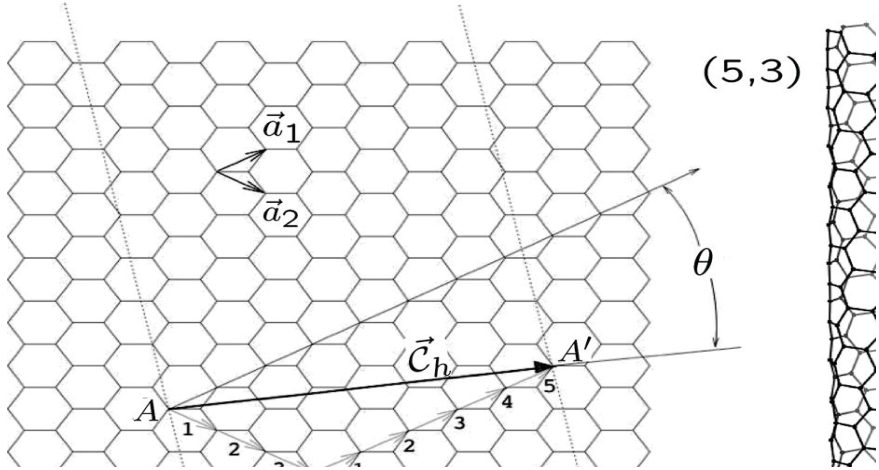
شكل رقم (٣-٢٣) أنبوب كربون نانوي من نوع chiral ناتج عن ثني لوح جرافيت (٤٥).
