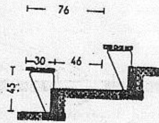
16 - على كتيفة معدنية مثبتة في البيتون
