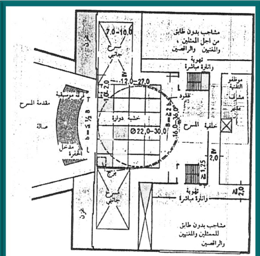
(5) مخطط تحليلي لمسرح بإبعاده العادية .
