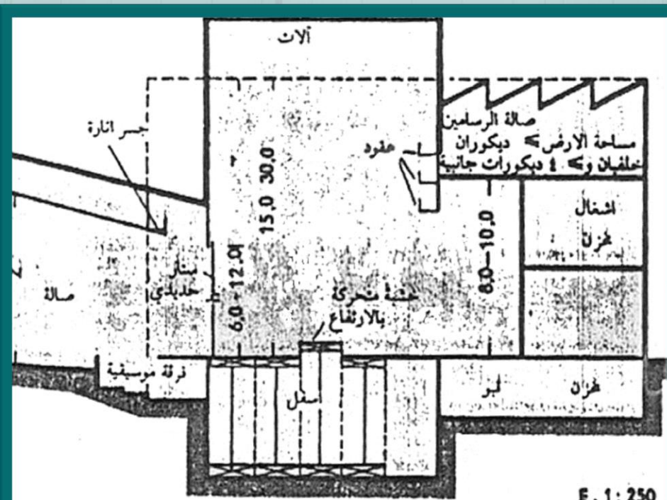
(6) مقطع تحليلي لمسرح : Z = الارتفاع الوسطي للصانة h = ارتفاع فتحة المسرح .
