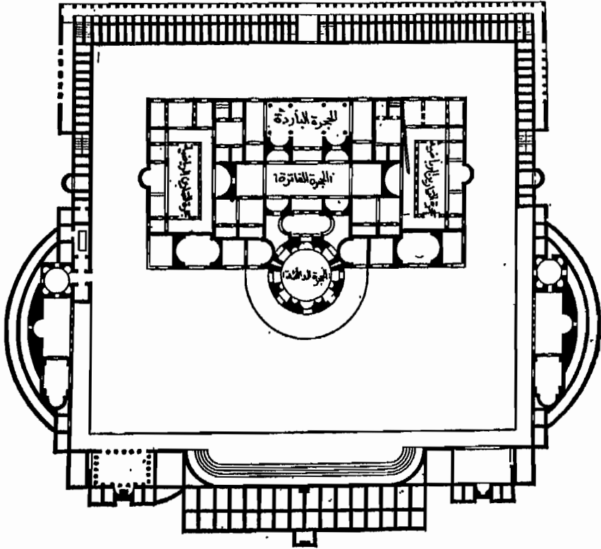
الشكل ٢٥ - حمامات كركلا
