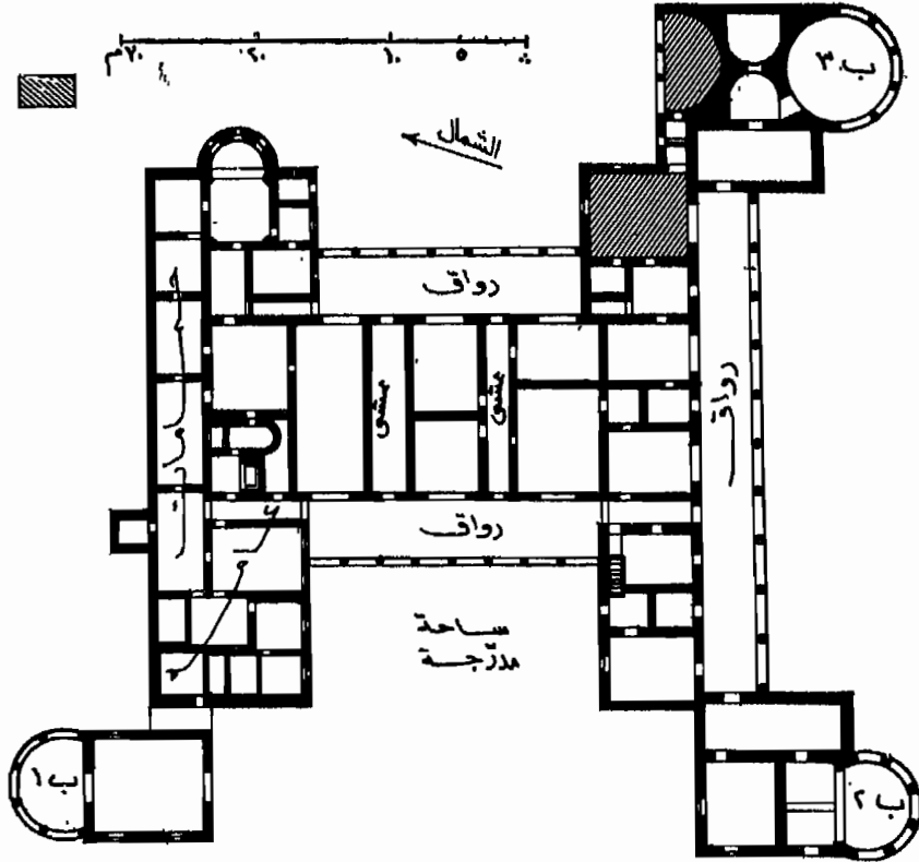
الشكل ٢٣ - « مقصف » اودرانغ شمالي تريف ب ١ - المدخل؛ ب ٢ و ب ٣ - كشكان؛ كانت بعض أقسام المقصف، على الأقل، تستأجر طبقة عليوية.
