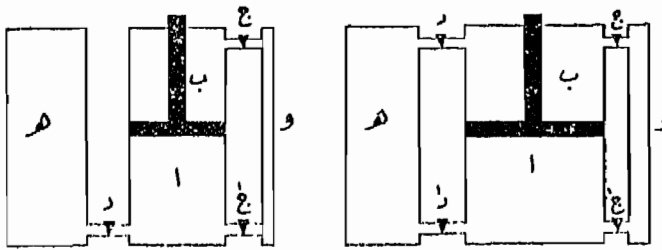
رسم الجاري لآلتي وات
