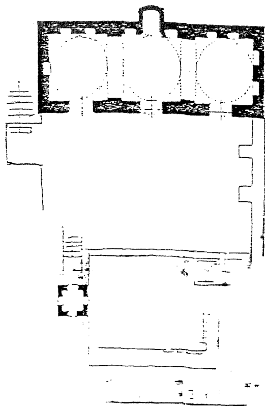
شكل (١٠٦) التحيطة ، مسجد الشيخ أ بكر ، المسقط الأفقى (ITALIAN INSTITUTE عن)
