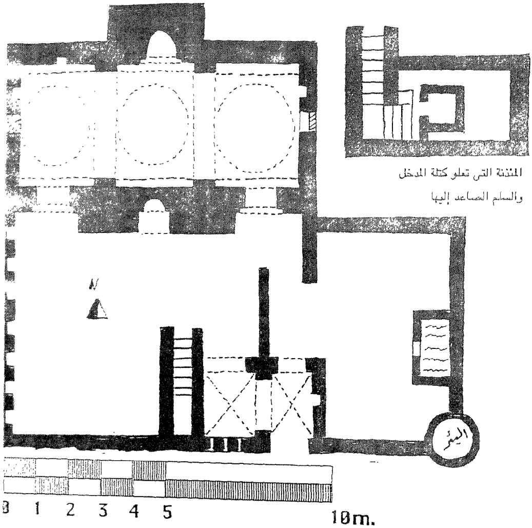
شكل (٤٨) حيس ، مسجد الموفى الأعلى ، المنقط الأفقى
