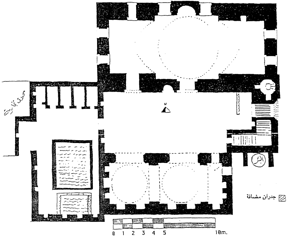
شكل (٧٧) حيس ، مدرسة الأسكندرية ، المسقط الأفقى
