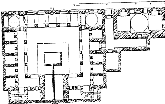
شكل (٩٣) ماردين ، المدرسة القاسمية ، المسقط الأفقى ( عن بريارا فنستر )
