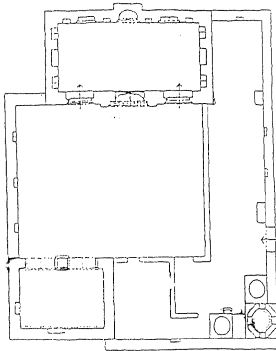
شكل (١٠٢) زبيد ، مسجد الصنوي ، المسقط الأفقي
