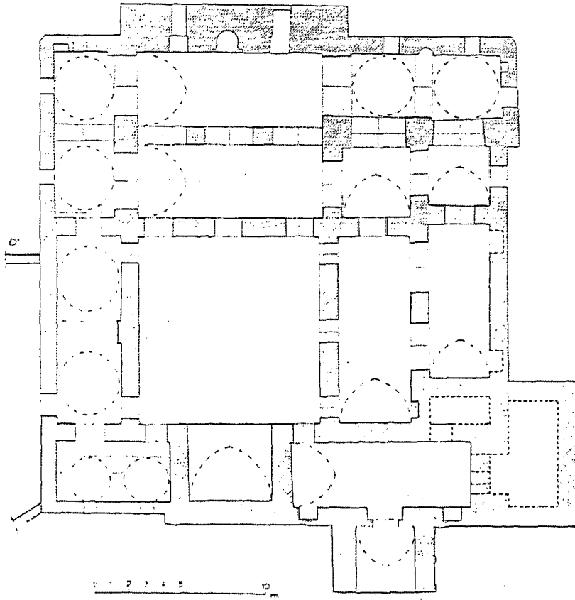
شكل (٨٥) حيس ، الجامع الكبير ، المسقط الأفقى كما وضعتة بربارا فنستر
