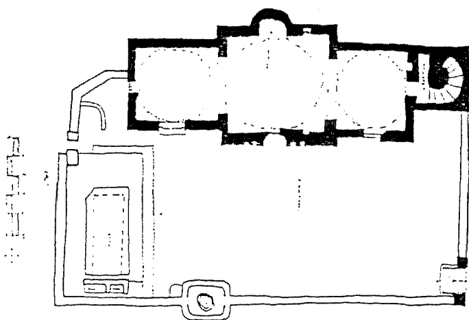
شكل (١٠٧) الدرهمى ، مسجد عبد الله بن على ، المسقط الأفقى (TEHAMAH عن)
