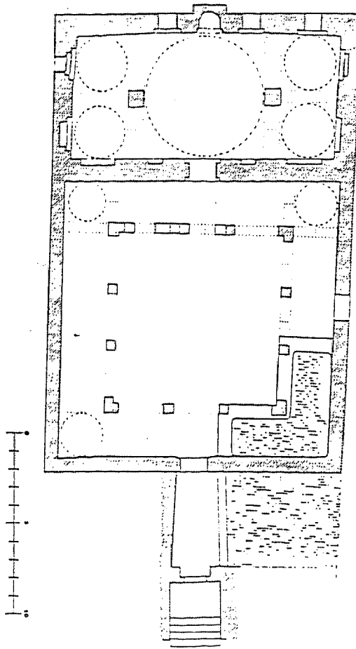
شكل (١١٧) إب، المدرسة الأسدية، المسقط الأفقى (عن بربارا فنستر)
