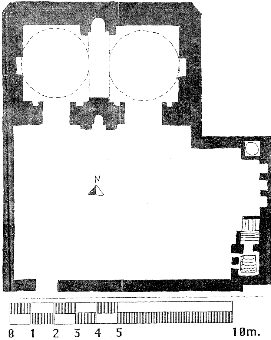
شكل (٣٢) حيس ، مسجد الكيلة ، المسقط الأفقى
