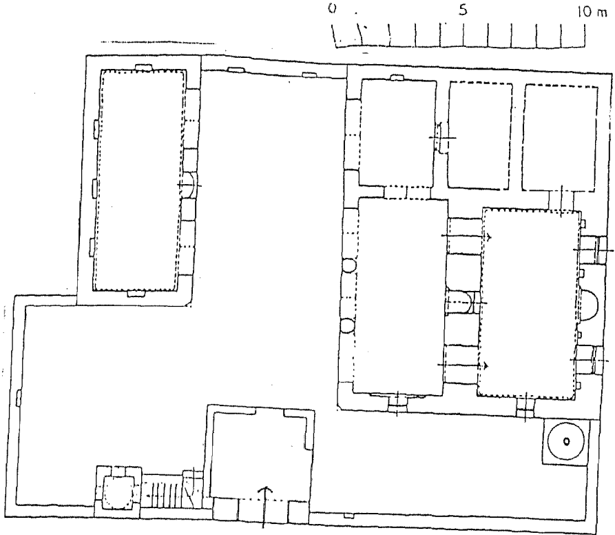
شكل (١١٣) زبيد ، مدرسة الرجاجي ، المسقط الأفقي (عن ITALIAN INSTITUTE)
