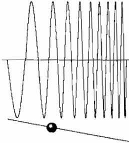
الشكل 7-8. الشكل العام لدالة موجية لخرزة تنزلق على سلك يميل بزاوية على الخط الأفقي، لذا يكون لها طاقة كامنة أخفض باتجاه اليمين. لاحظ أن طول الموجة يُقصرُ حين نسير باتجاه اليمين، وهذا يقابل تقليدياً الطاقة الحركية المتزايدة للجسيم خلال انزلاقه إلى الأسفل على السلك.
