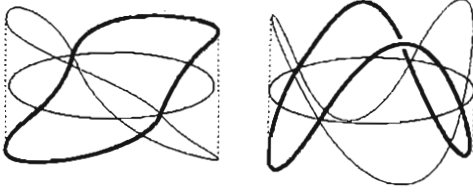
الشكل 6-15. نمطان للاهتزازِ صغريّ النقطيّة لوتر، ويقابل كلُّ نمطٍ منهما جسيمٌ أوليٌّ مختلفٌ عما يمثله النمطُ الآخر.
