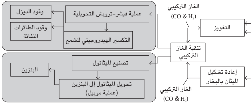
شكل ٦-١: صنع الوقود السائل عن طريق الغاز التركيبى.
