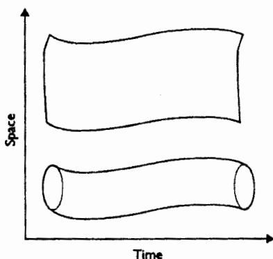
شكل (٤-٣) عندما يتحرك وتر مفتوح النهاية فى الفضاء المكانى - الزمانى، فإنه يرسم سطحاً مستوياً. بينما الوتر المغلق النهاية يرسم أنبوباً.
