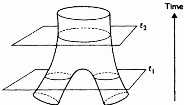
شكل (٤-٥) الأوتار المغلقة يمكنها الاندماج معاً حيث يندمج وتران مغلقان لتكوين وتر ثالث ويطلق على الشكل شكل البنطلون.
