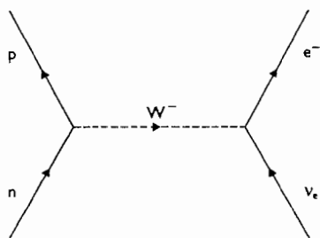
شكل ٢-٤ جميع التفاعلات الأساسية يمكن تمثيلها بواسطة مخطط فينمان. فى هذه الحالة المخطط يمثل انحلال بيتا على مستوى النيوترون والبروتون.
