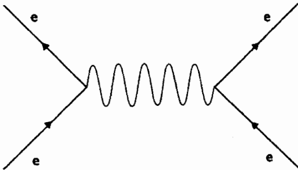
شكل (٢-٢) شكل فينمان التقليدى لتفاعل الجسيمات - فى هذه الحالة يتفاعل إلكترونان مع بعضهما عن طريق تبادل فوتون.
