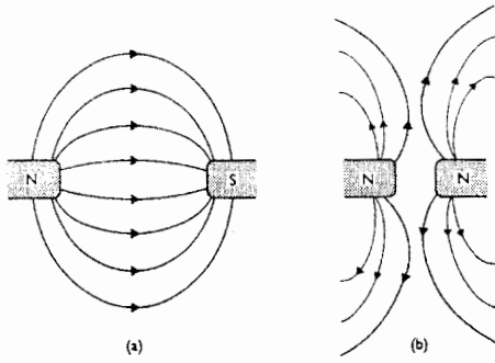
شكل (٢-١) فكرة خطوط القوى والتي ابتكرها فاراداي تفيد في توضيح كيف تتنافر الأقطاب المغناطيسية المتشابهة وتتجاذب الأقطاب المغناطيسية المختلفة.
