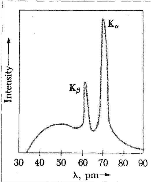
الشكل (11-1) طيف الأشعة السينية.
