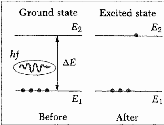
الشكل (10 - 1) يوضح عملية الامتصاص التحريضي.
