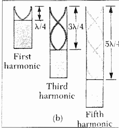
الشكل (14- 2) حالات الرنين في الأعمدة الهوائية المغلقة.
