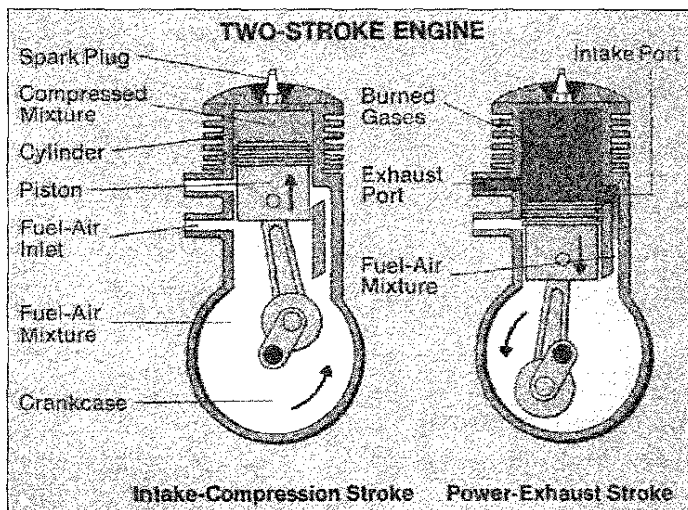
الشكل (15 - 12) محركات ذات دورة من ضربتين
