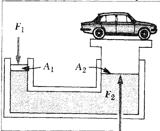
الشكل (3- 1) المكبس السوائلي
