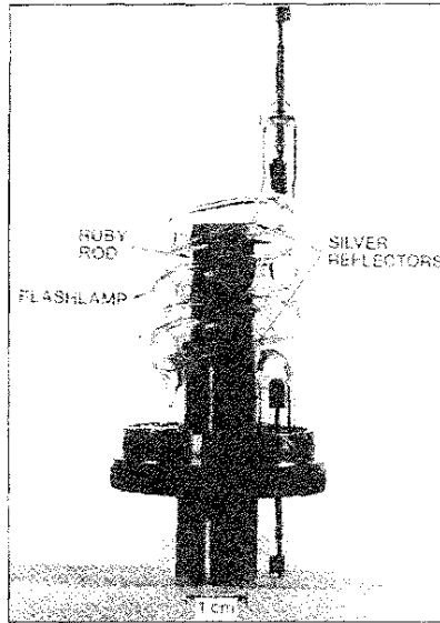
الشكل رقم (10 - 4): أول ليزر تم تطويره
