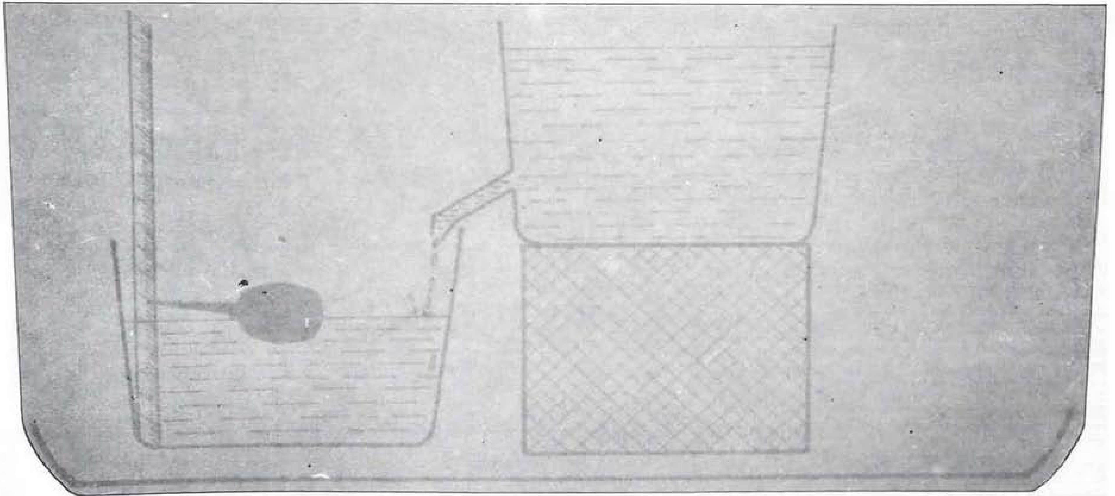
رقم (٢٠٩) ص ٣٢٣ ساعة الصنهاجي - القرمطوني المائية (٥٧١٧) كما تصورها الدكتور بدرون . هناك ظرف كبير يحتوي الحوضين معا : الحوض الايمن الذي وضع على دكة ، يتخذ منه الماء بقدر معلوم الى الحوض الايسر حيث يوجد عائم يطفو مؤشرا على مسطرة منتصبة هناك فيها البروج والشهور الفلاحية والساعات والدقائق .
