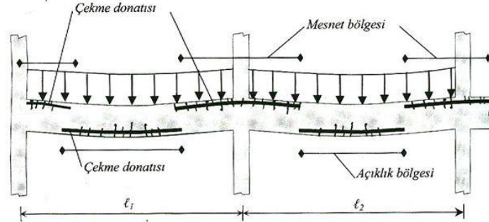
(a) Sürekli kiriş ve şematik olarak sehim yapmış durumu
