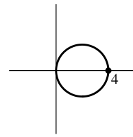
24. Circle
