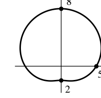
35. Limaçon
