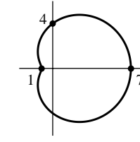
32. Limaçon
