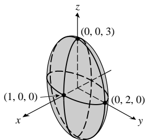
15. Ellipsoid
