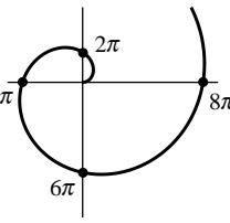
40. Spiral
