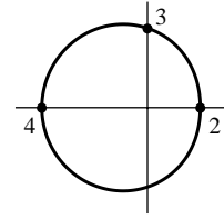
17. Limaçon
