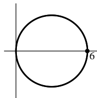
14. Circle
