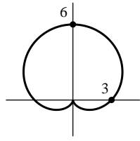
27. Cardioid
