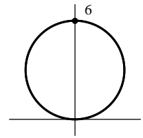
25. Circle
