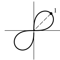
16. Lemniscate
