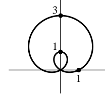
30. Limaçon
