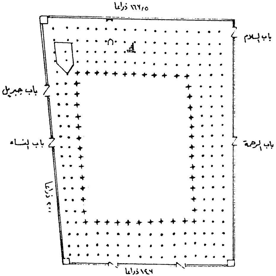
(شكل ٩) : مسقط أفقى للمسجد النبوي الشريف عقب عمارة الوليد بن عبد الملك . عن محمد هزاع الشهرى.
