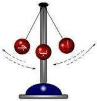
البندول البسيط
