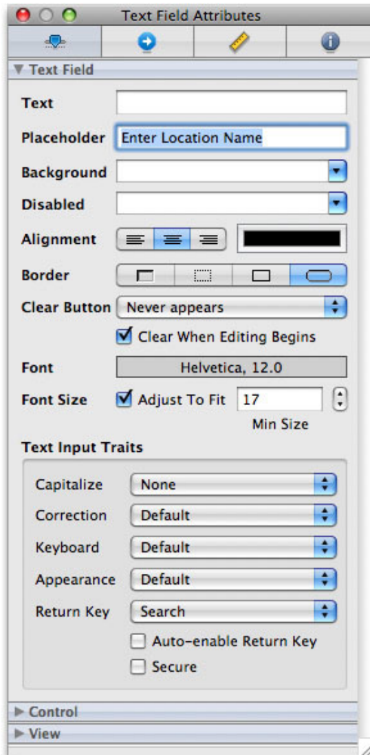
Figure 5.4. UITextField attributes
