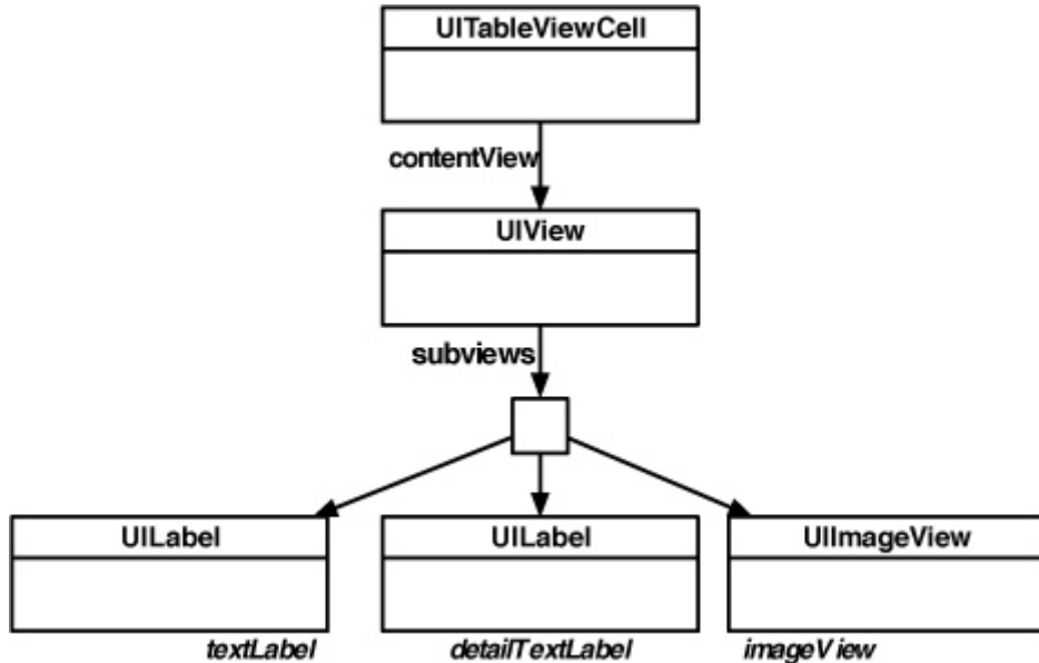
Figure 10.12. UITableViewCell hierarchy
