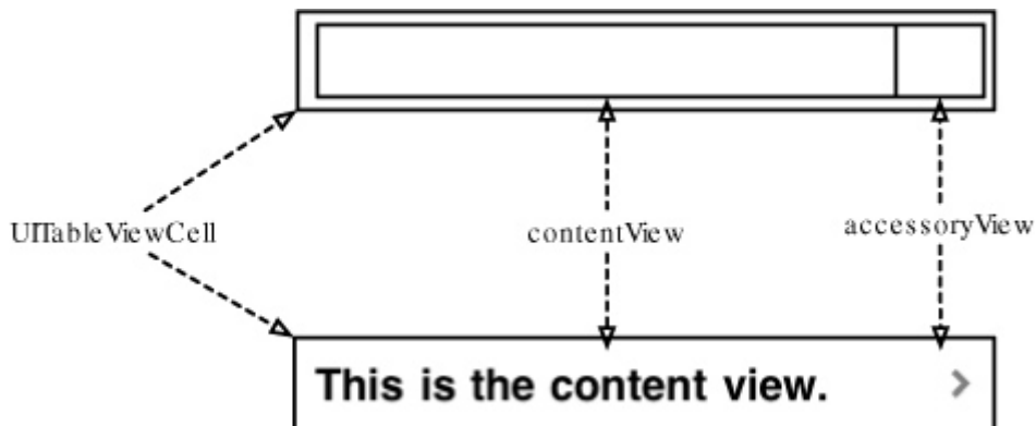
Figure 10.11. UITableViewCell layout
