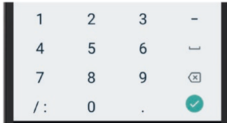
Figure 4-6. TextInputType.datetime
