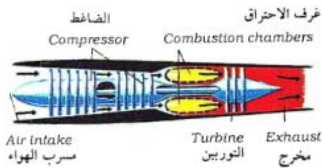
Turbojet engine محرك نفاث
