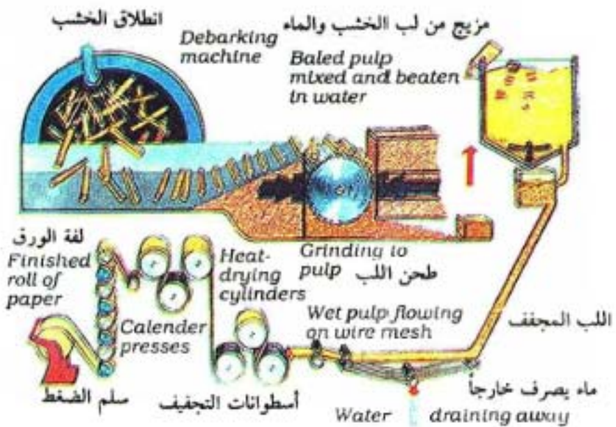
This diagram shows how paper is made from wood. رسم يبين كيفية صنع الورق من الخشب
