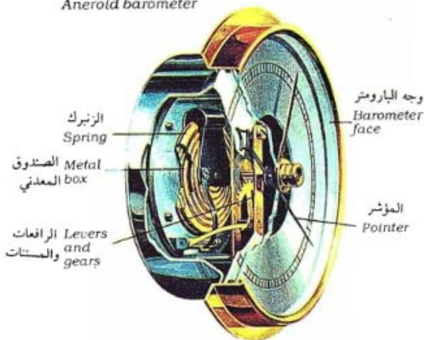
البارومتر المعدني Aneroid barometer
