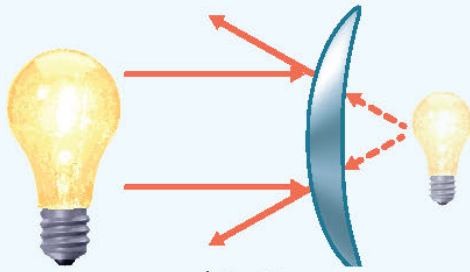
مرآة محدبة
