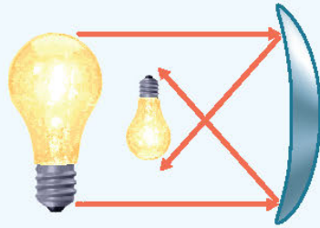
مرآة مقعرة
