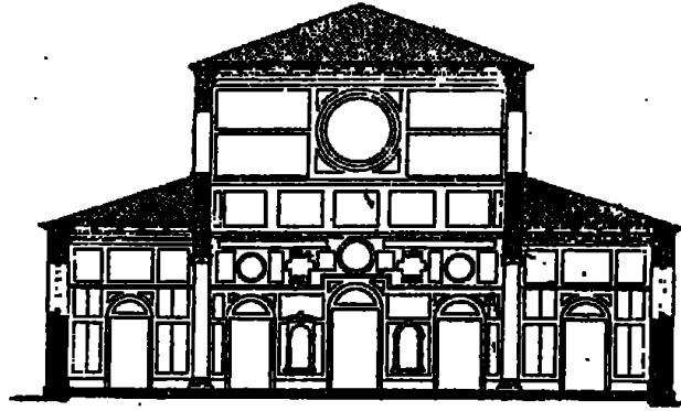
قطاع رأسى في كنيسة بازيليسكية
