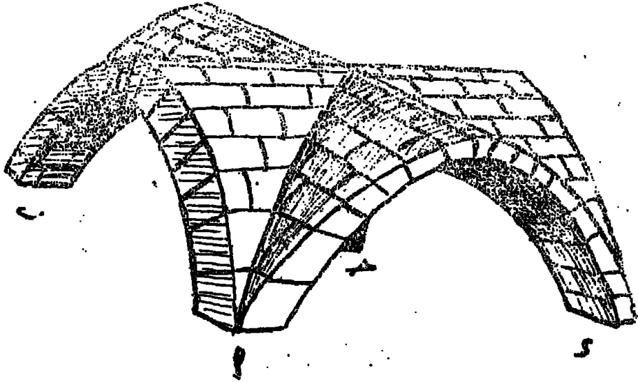
رسم تخطيطي يوضح إقامة السقف الحجري على شكل أقواس تحملها عمد
